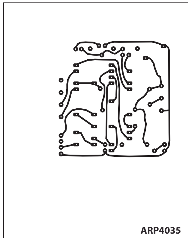
Top Foil
