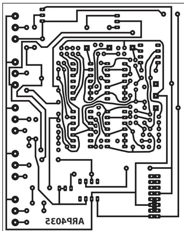
Bottom Foil
